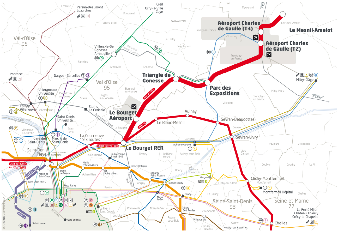
Figura 2.23 Grand Paris Express: opere del quadrante nord
