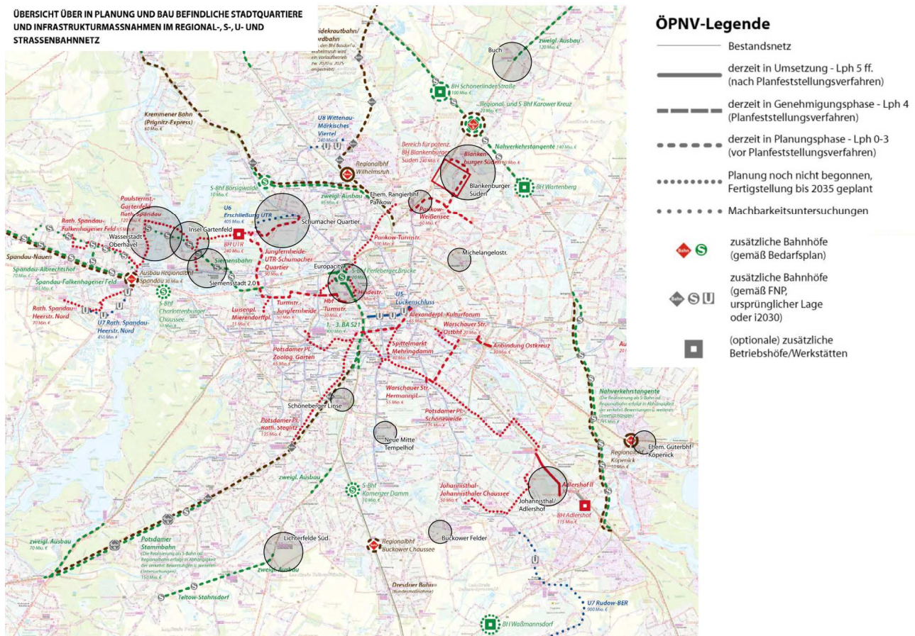
Figura 2.42 Interventi di ampliamento della rete U+S Bahn e miglioramento dell'impedenza del nodo verso l'attraversamento della città da parte dei servizi suburbani e regionali.
