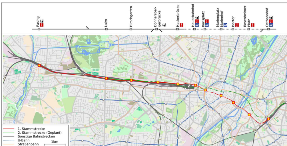
Figura 2.44 Il passante ferroviario di Monaco (S-Bahn-Stammstrecke München) è costituito da una sede riservata per i servizi S-Bahn 11,4 km la cui parte principale è la galleria di 4,3 km completata nel 1972. Dal 2017 è iniziata la costruzione del quadruplicamento della galleria (in basso), i cui lavori dovrebbero terminare nel 2028
