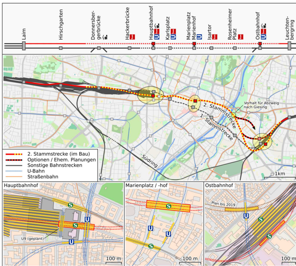
Figura 2.44 Il passante ferroviario di Monaco (S-Bahn-Stammstrecke München) è costituito da una sede riservata per i servizi S-Bahn 11,4 km la cui parte principale è la galleria di 4,3 km completata nel 1972. Dal 2017 è iniziata la costruzione del quadruplicamento della galleria (in basso), i cui lavori dovrebbero terminare nel 2028
