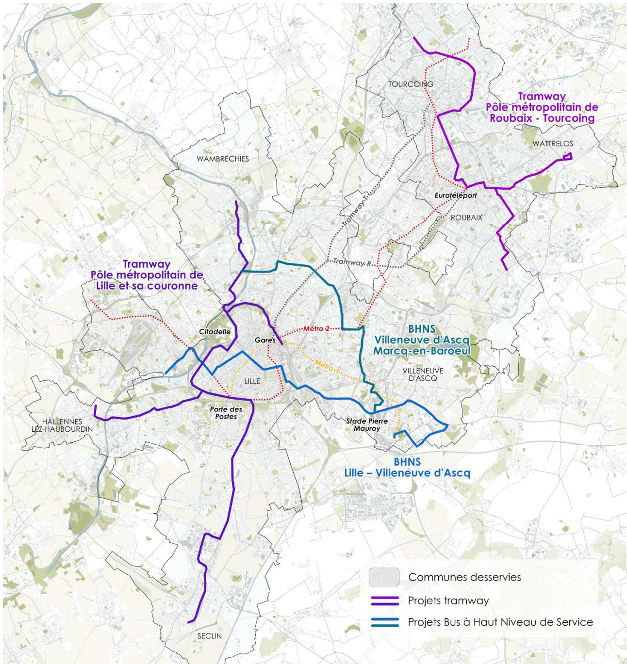
Figura 2.32 Città metropolitana di Lilla: Schema direttore del trasporto rapido incentrato su una nuova rete tranviaria (in viola), 5 linee a integrazione della storica Y (in grigio scuro) per Tourcoing e Roubaix, da completare entro il 2035
