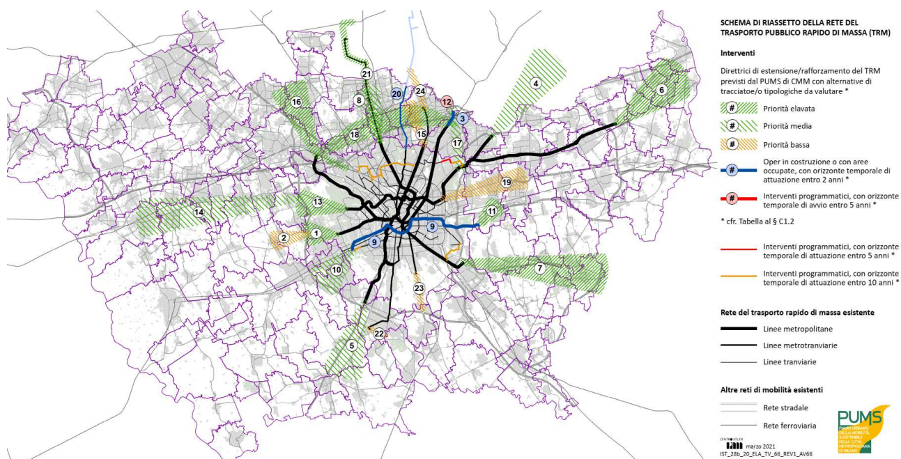
Figura 2.104 PUMS, interventi sulla rete del trasporto rapido di massa
