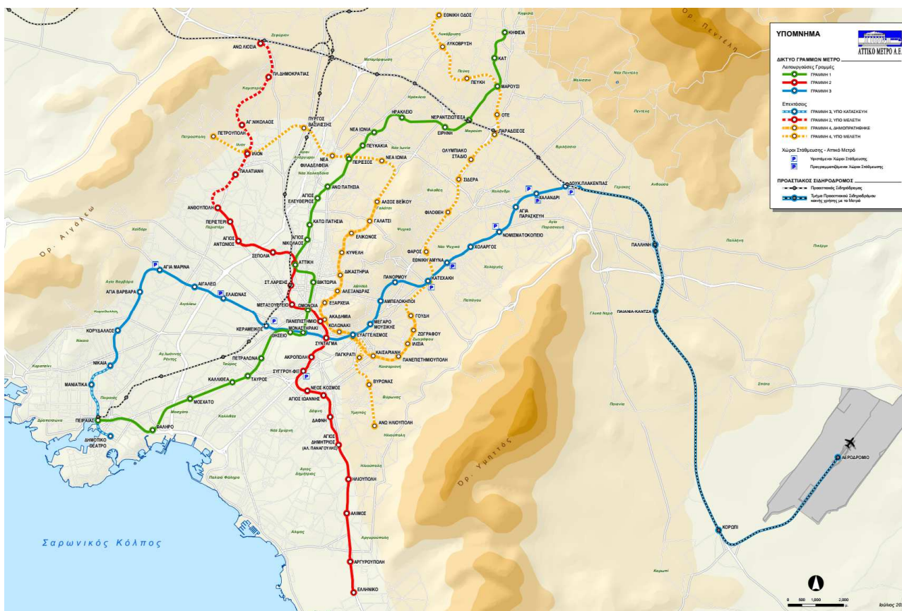
Figura 2.55 Atene, rete metropolitana esistente e nuova linea 4 (in giallo)
