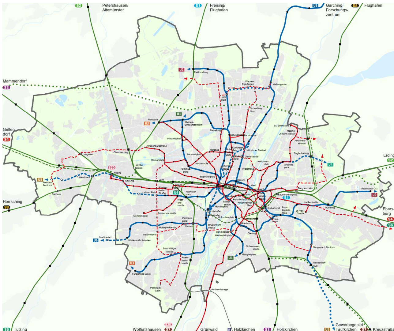
Figura 2.45 Piano di ampliamento del trasporto rapido di massa: in blu le U-Bahn (metro), in verde le S-Bahn (linee ferroviarie suburbane), in rosso le tranvie
